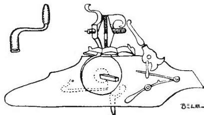
Roda de arcabuz com a manivela
